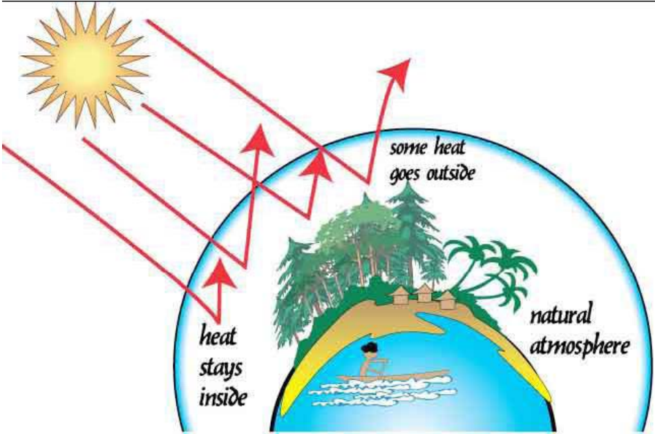
השמש: מקור האנרגיה העיקרי של כדור הארץ
